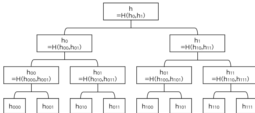
図表 A-2：マークル木の構造
