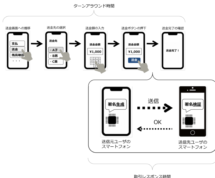
図表 3：電子現金処理にかかる操作
