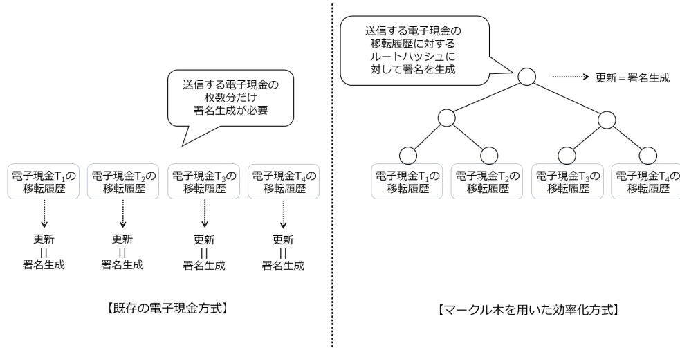
図表 7: マークル木を用いた効率化方式
