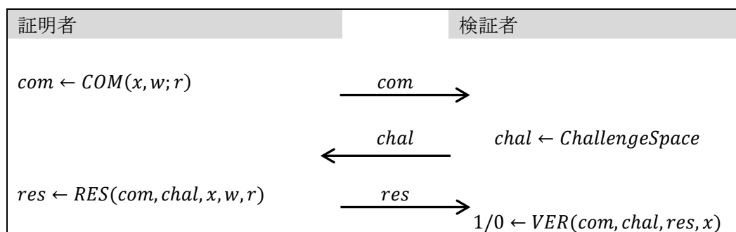
図表 A-3 : \Sigma プロトコル
