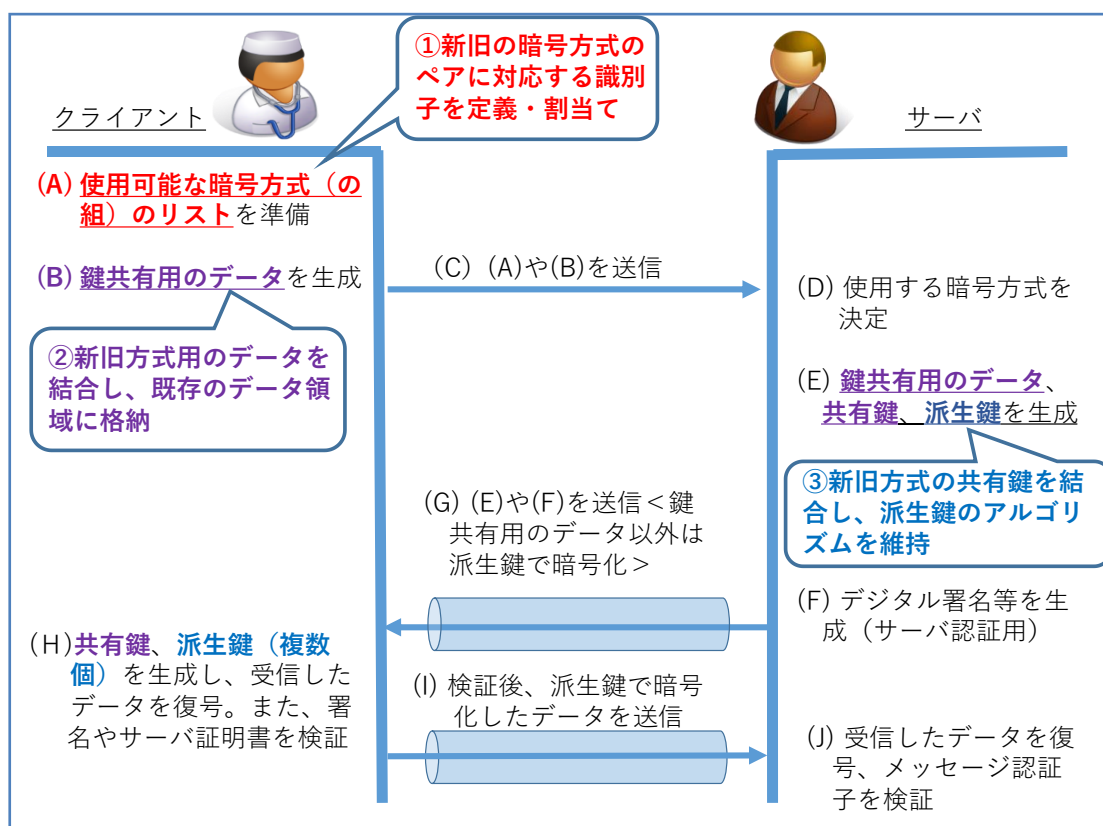
図表 2 TLS 1.3 における鍵共有部分の仕様拡張のイメージ
