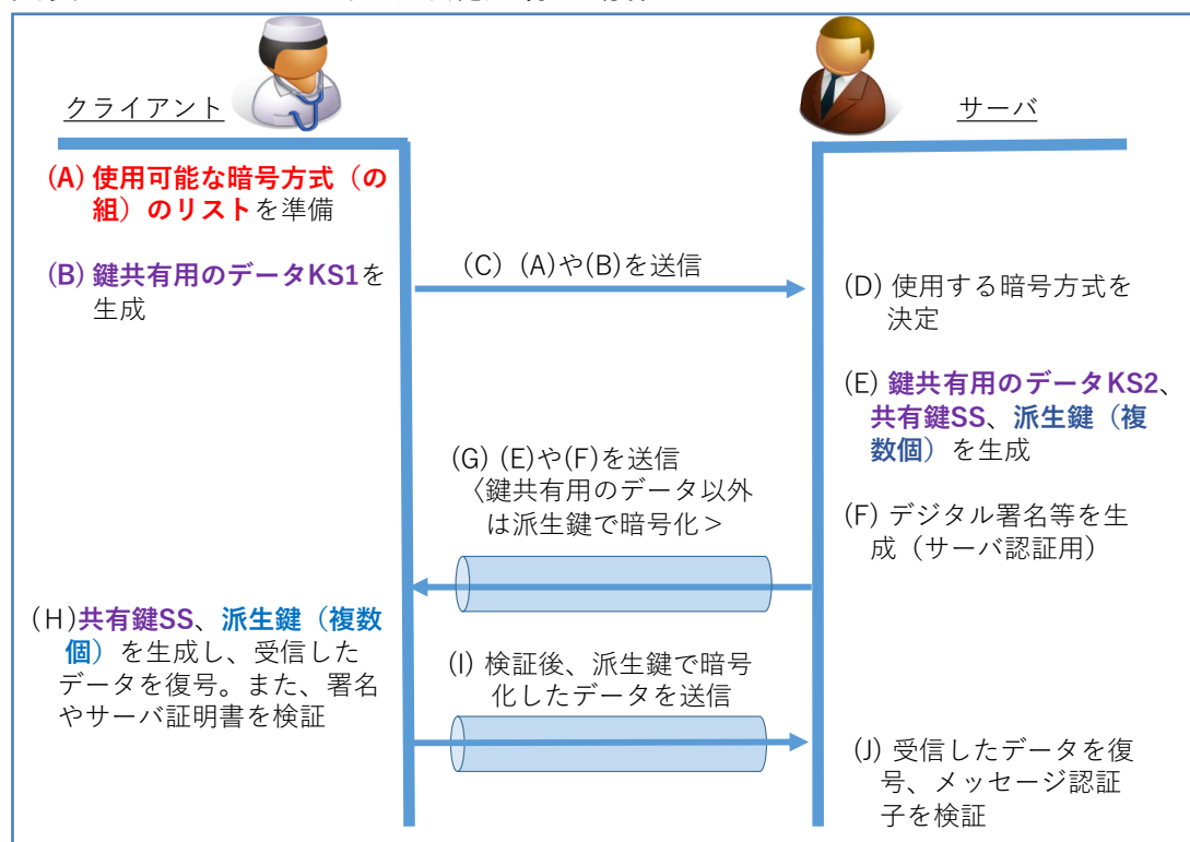
図表 A-1 TLS 1.3 における鍵共有の動作のイメージ
