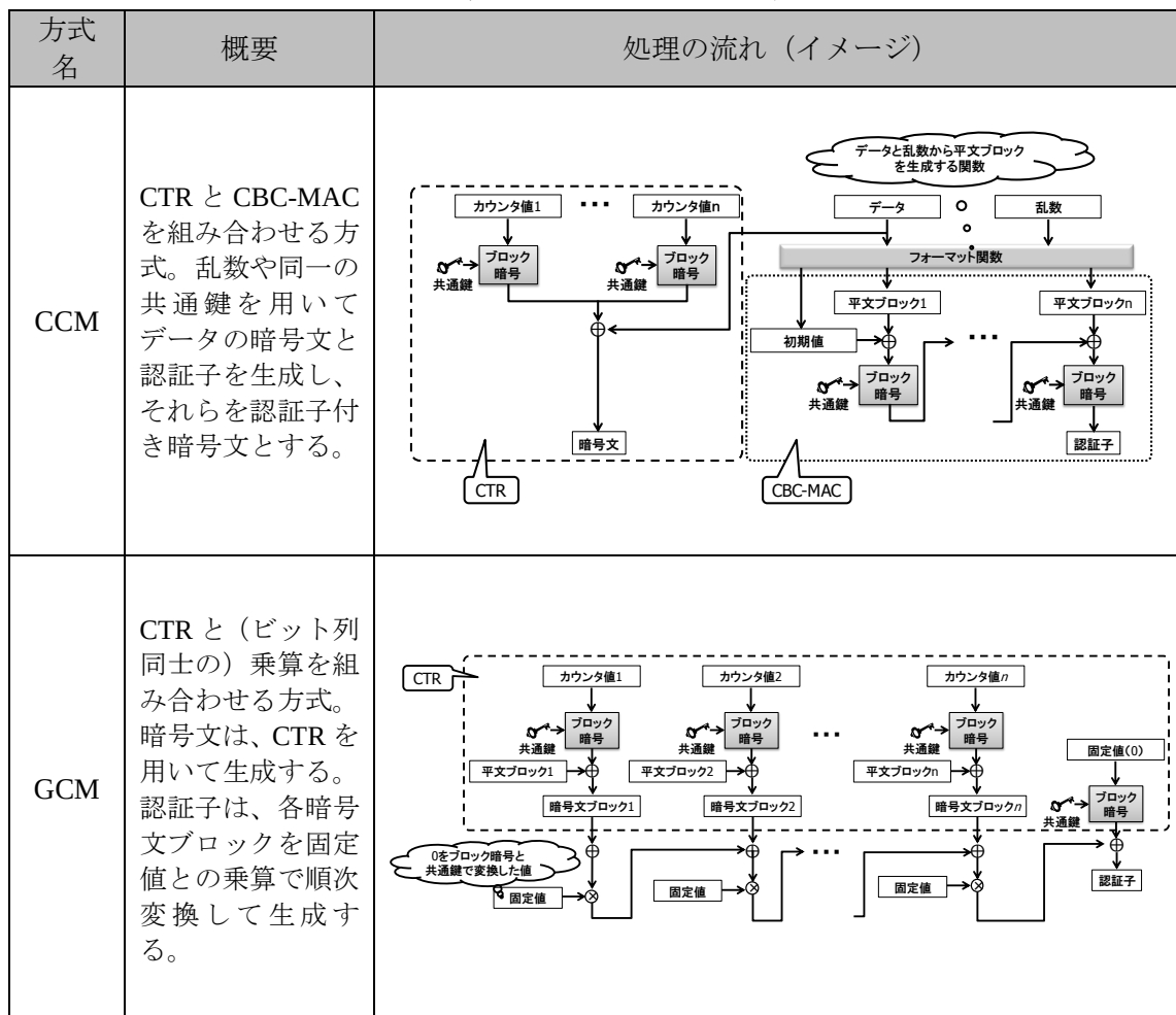
図表 4. 認証付き秘匿機能を実現する暗号利用モード
