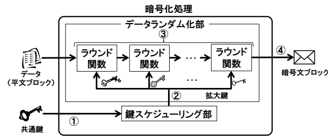
図表 1. ブロック暗号の典型的な暗号化処理
