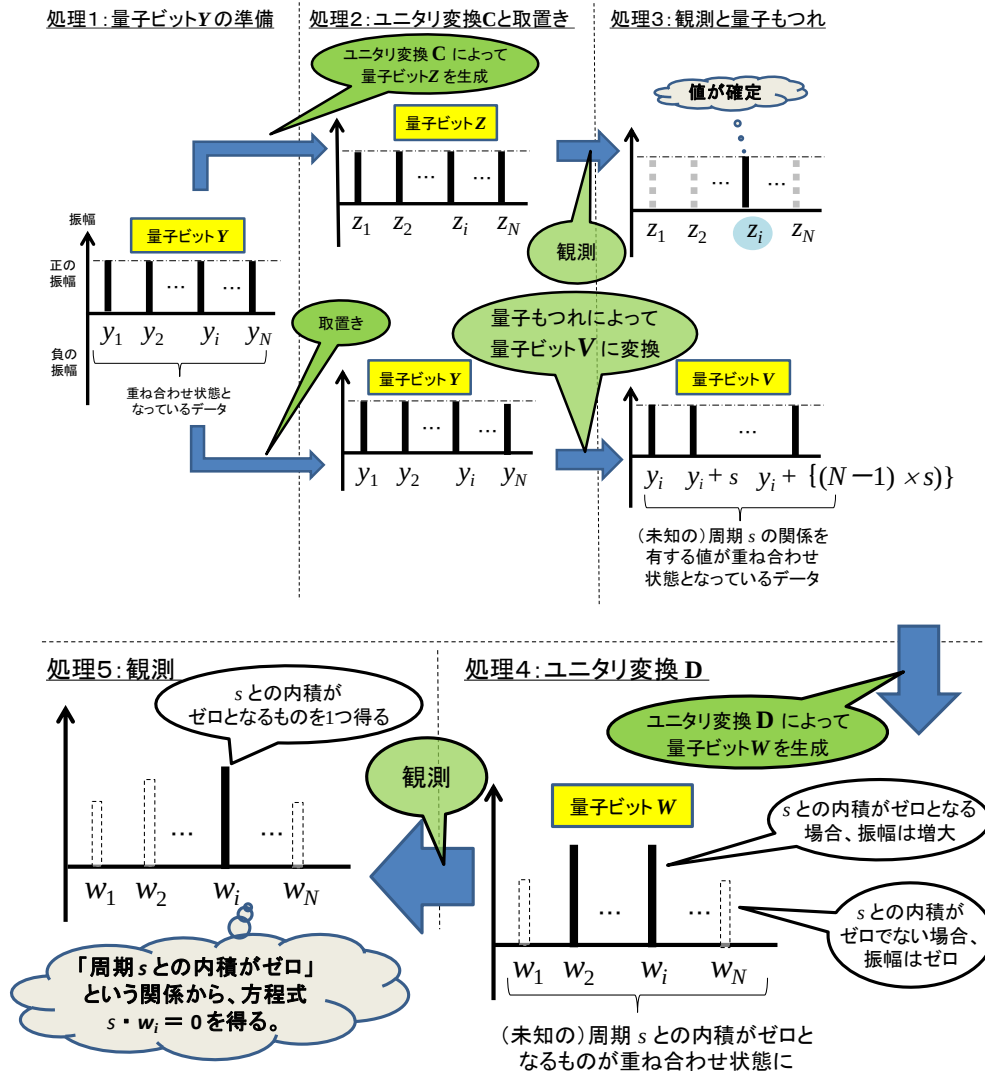
図表 7. サイモンのアルゴリズム (イメージ)
