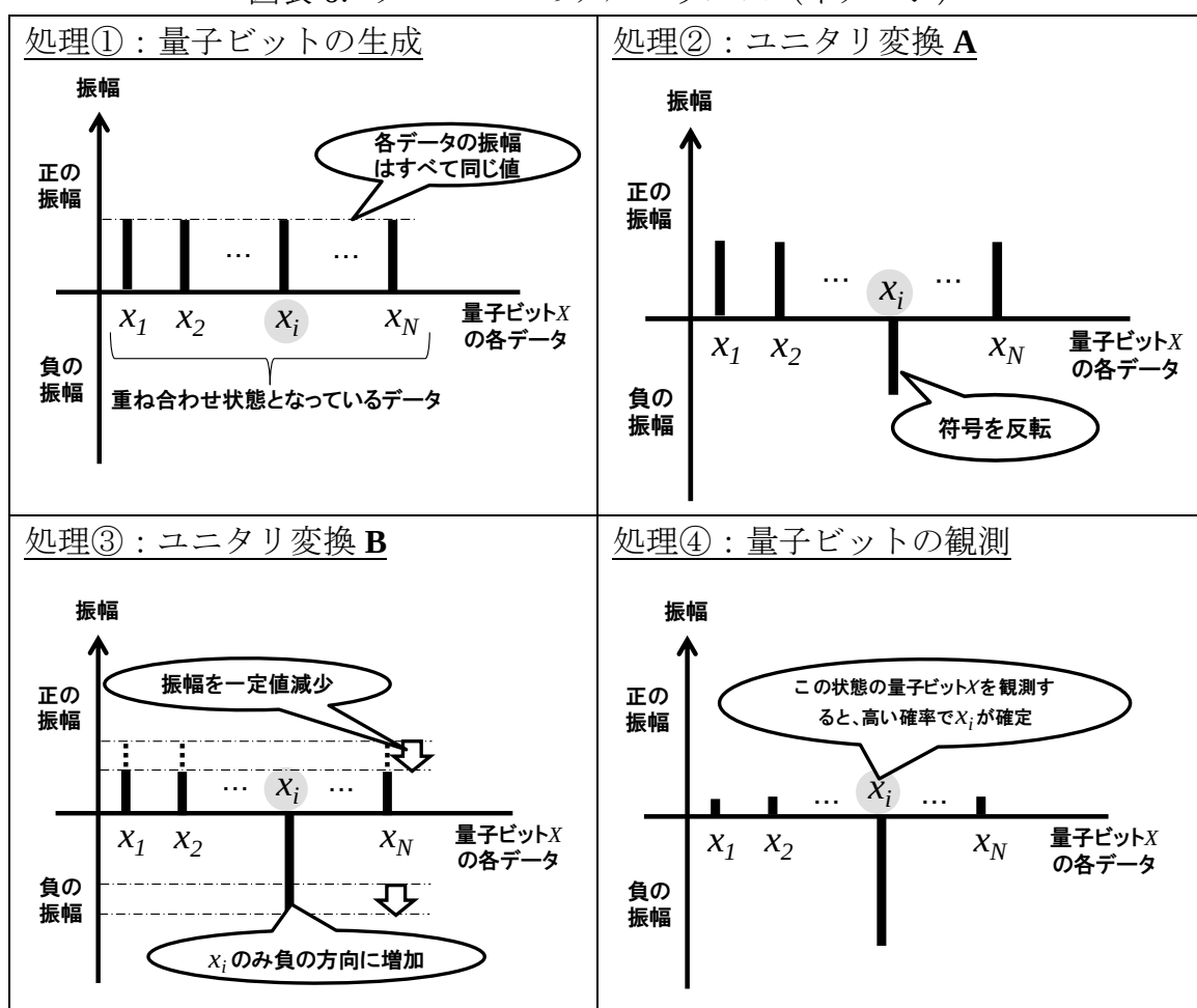
図表 6. グローバーのアルゴリズム（イメージ）
