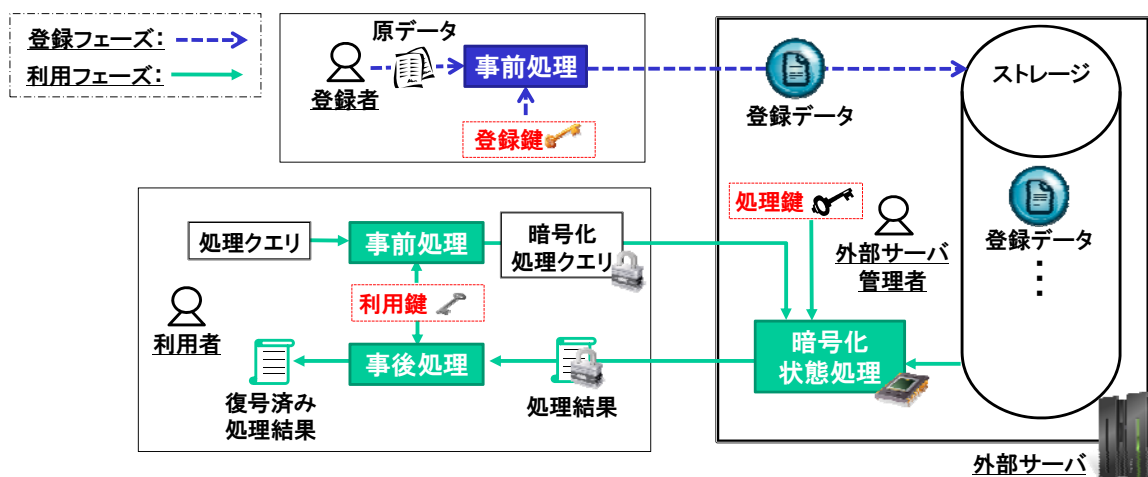
図表 3. 登録データの登録・利用に関する処理フロー
