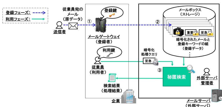
図表6. 秘匿検索の電子メールシステムへの応用例
