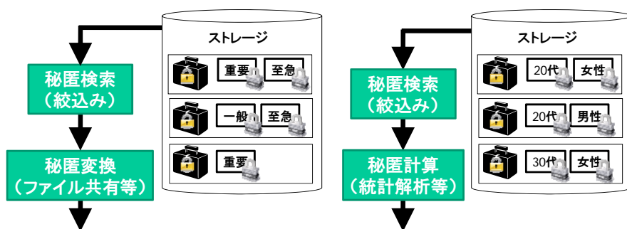
(a) 秘匿変換との組合せ (b) 秘匿計算との組合せ
