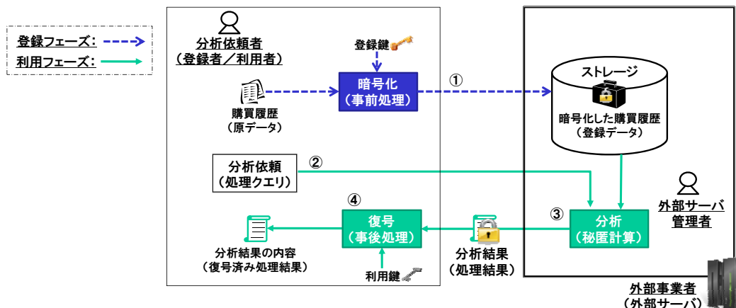
図表 18. 秘匿計算のデータ分析委託サービスへの応用例
