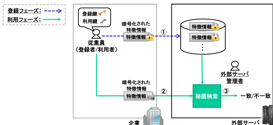
図表 7. 秘匿検索の生体認証システムへの応用例
