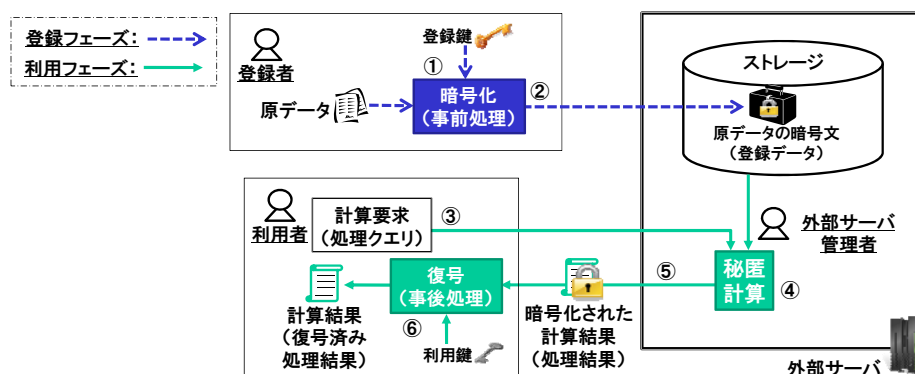
図表 17. 秘匿計算の処理フロー
