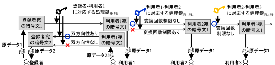
図表 14. 秘匿変換の2つの変換機能
