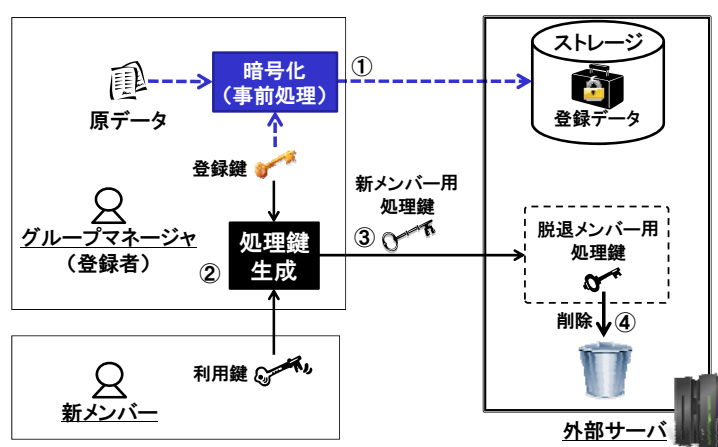
図表 12. 秘匿変換のファイル共有システムへの応用例
