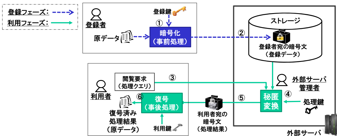
図表 10. 秘匿変換の処理フロー
