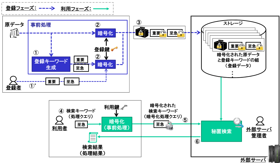
図表 5. 秘匿検索の処理フロー
