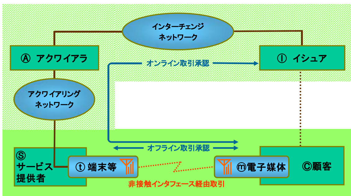
図1 一般化したリテール取引システムの全体イメージ（例） と非接触インタフェース利用箇所
