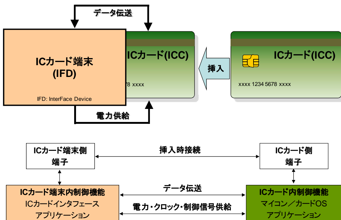
図2 ICカード(端子付き)の内部構造イメージ
