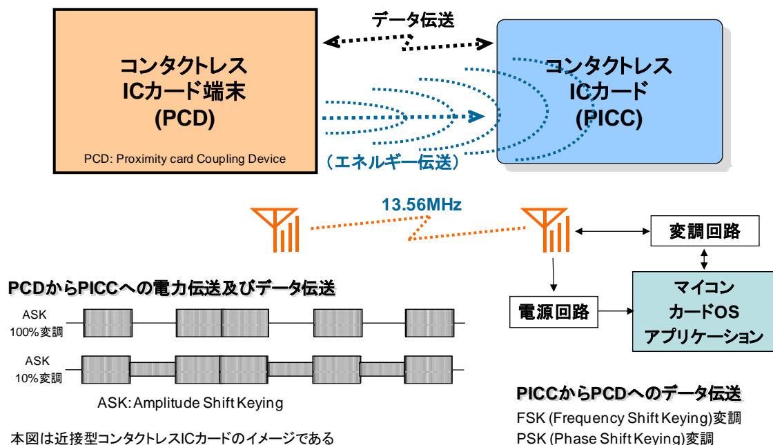
図3 コンタクトレス IC カードの内部構造イメージ
