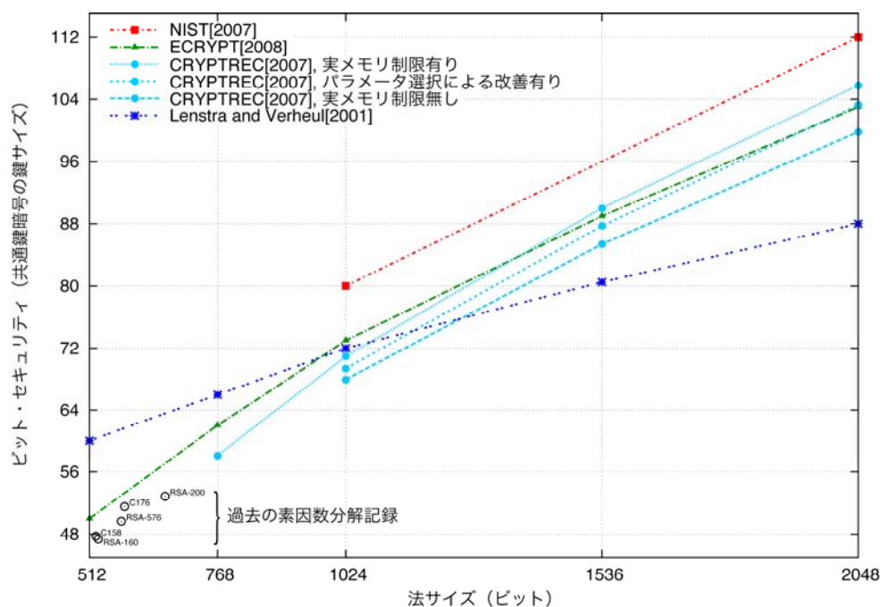
図表 A2：一般数体ふるい法での計算量において等価な法サイズと共通鍵暗号の鍵サイズの推定
