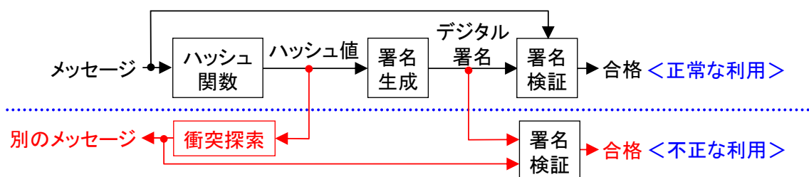
図表 2：デジタル署名におけるハッシュ値の衝突を使った攻撃例
