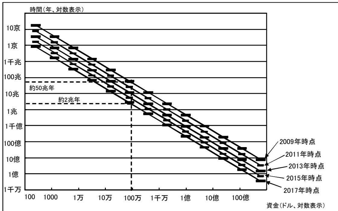
図表 4 : 128 ビットの鍵の全数探索に必要な資金と時間の関係
