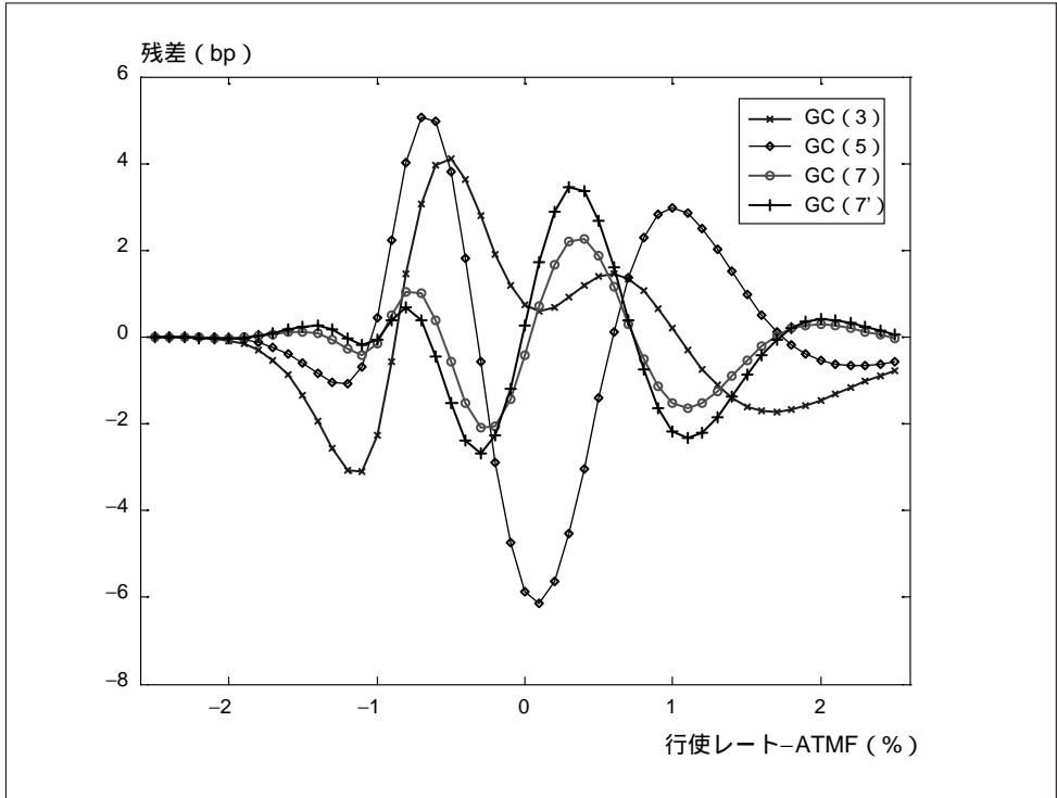
図9 「1 into 10スワップション」のGC展開による価格の残差(CIRモデル)
