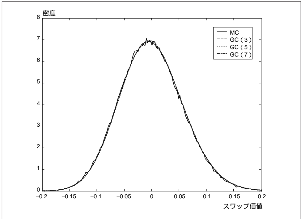
図3 1年後の10年スワップの価値の密度関数(ガウシアン・モデル)
