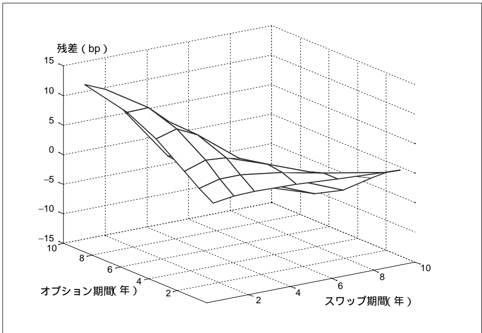
図10 スワップションのGC(7)による価格の残差(CIRモデル)
