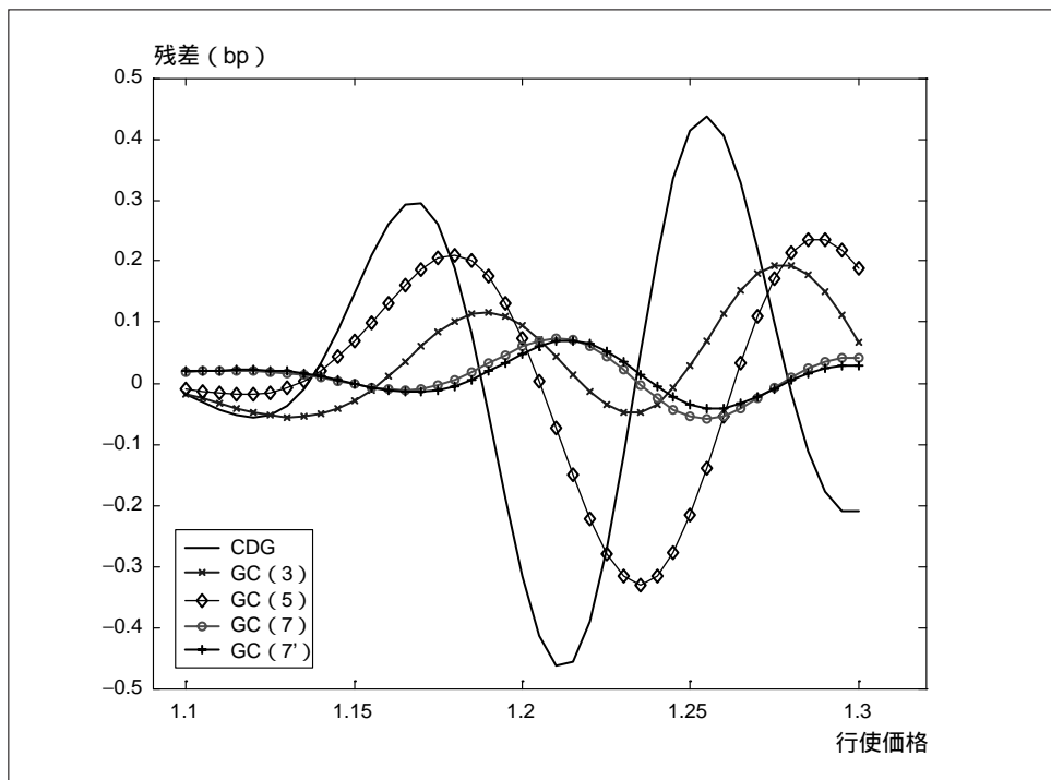
図11 スワップションのGC展開とCDGによる価格の残差 (CIRモデル)
