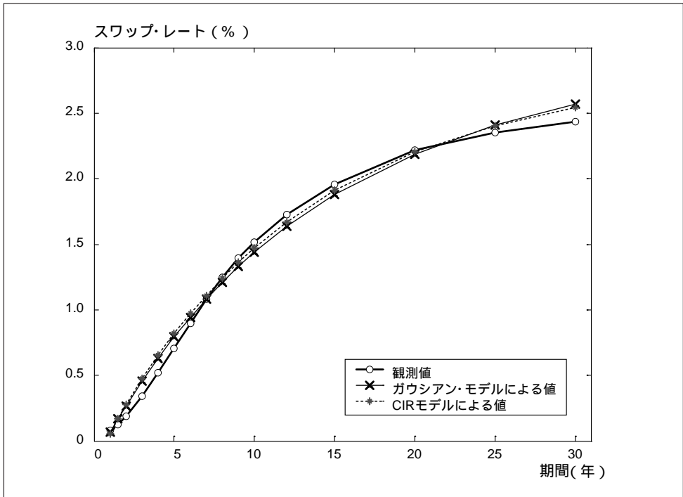
図1 スワップ・レートの観測値とモデルによる値
