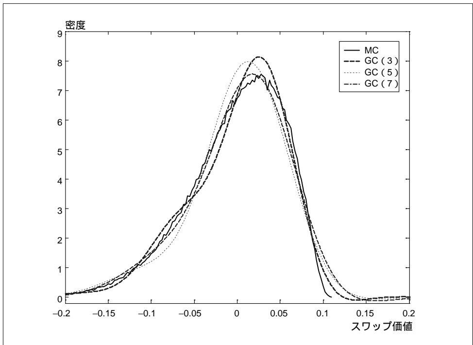
図4 1年後の10年スワップの価値の密度関数(CIRモデル)
