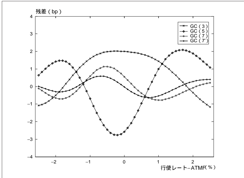
図7 「5 into 10スワップション」のGC展開による価格の残差(ガウシアン・モデル)
