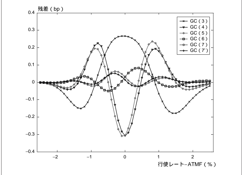
図5 「1 into 10スワップション」のGC展開による価格の残差(ガウシアン・モデル)
