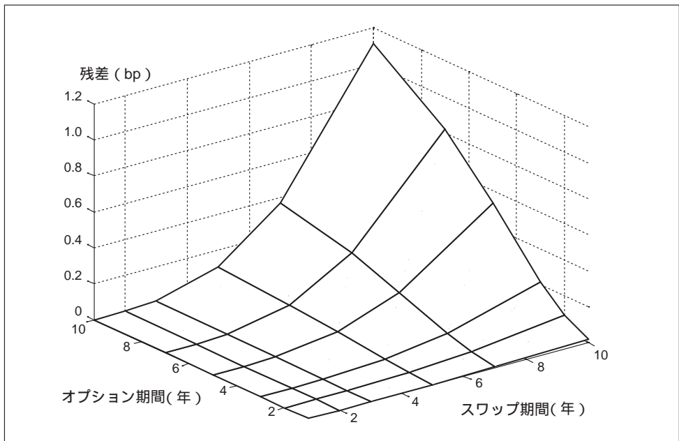
図8 スワップシヨンのGC(7)による価格の残差(ガウシアン・モデル)
