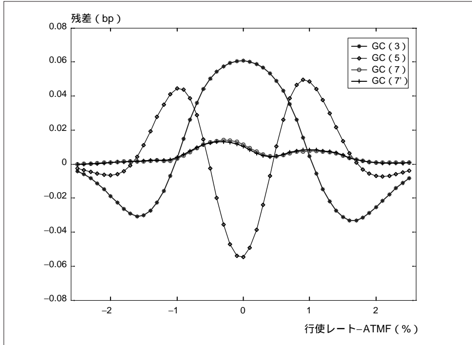
図6 「1 into 5スワップション」のGC展開による価格の残差(ガウシアン・モデル)
