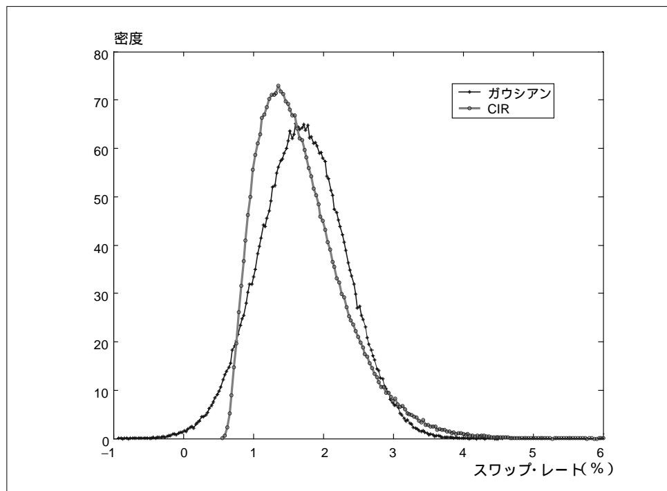
図2 MC法による1年後の10年スワップ・レートの密度関数
