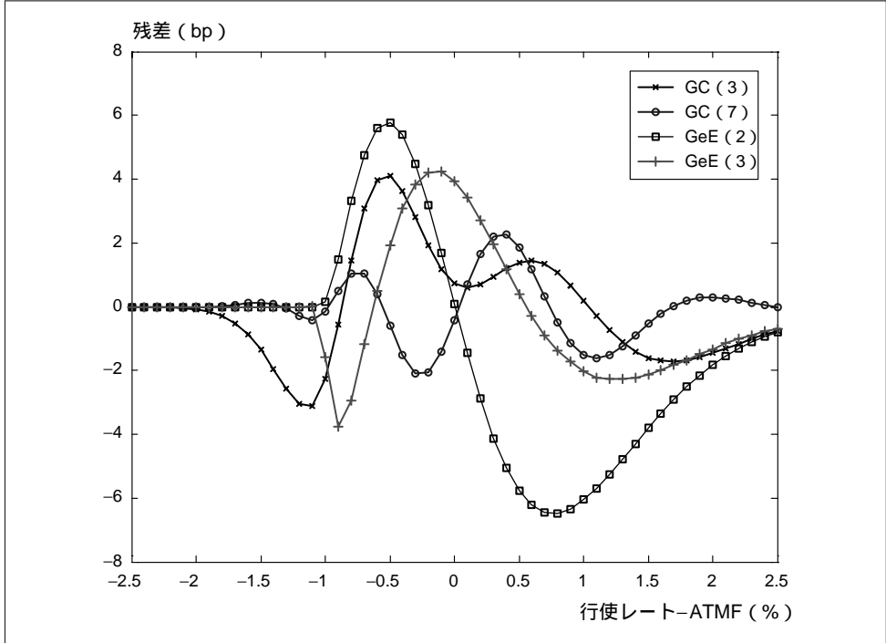
図12 「1 into 10スワップション」のGC展開とGeE展開による価格の残差 (CIRモデル)
