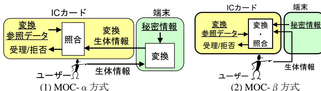
図表 10. 類似度保存アプローチを適用した生体認証システムの例
