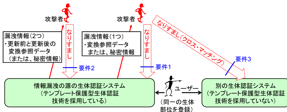
図表 7. テンプレート保護型生体認証技術の主なセキュリティ要件
