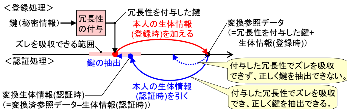
図表 9. 鍵抽出アプローチにおける基本アイデア
