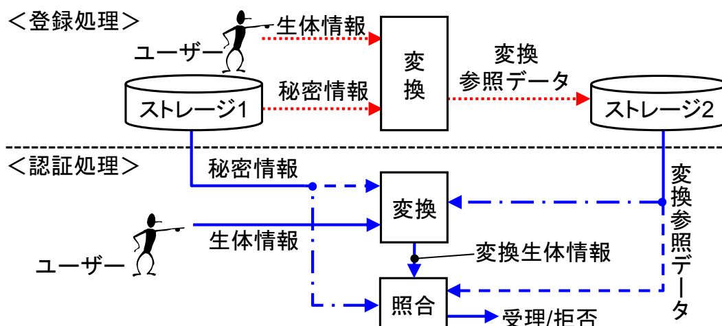
図表 6. テンプレート保護型生体認証の処理フロー（概念図）
