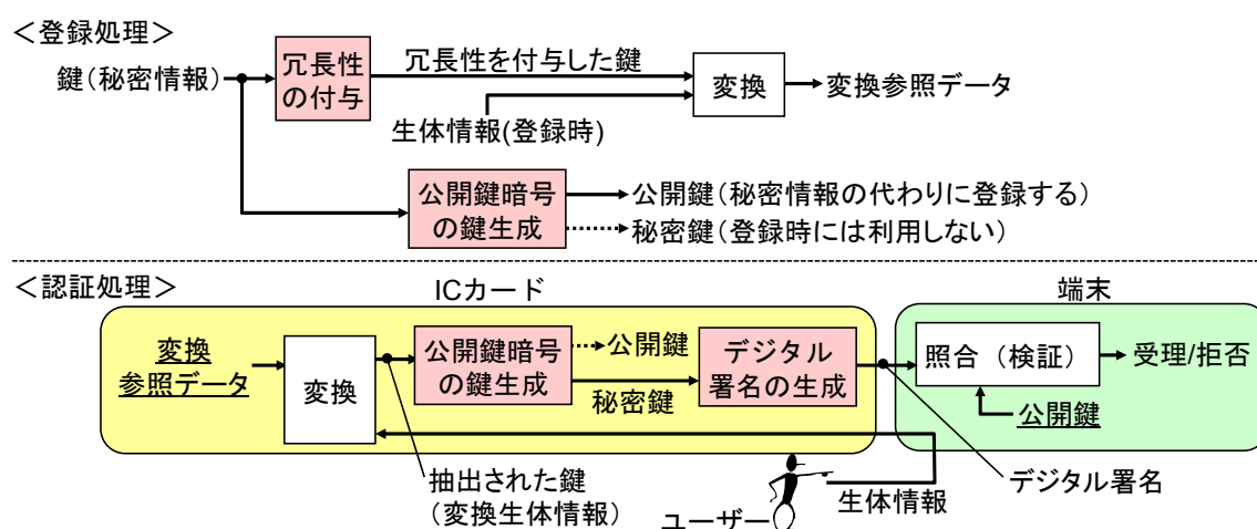
図表 B-1. STOC- \alpha 方式の登録と認証の処理フロー
