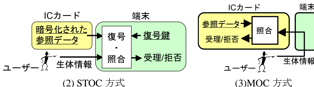
図表 2. STOC 方式と MOC 方式
