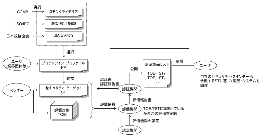
図 4：コモンクライテリアに基づくセキュリティ評価・認証の枠組み
