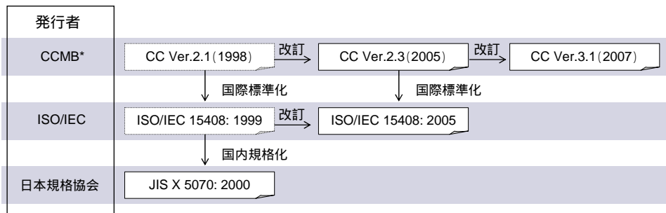
図 3 : CC、ISO/IEC 15408、JIS X 5070 の対応関係
